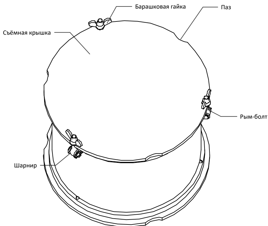
Рисунок 4 - Барабан
