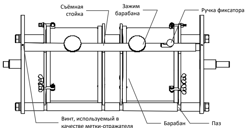
Рисунок 5 – Держатель барабанов
