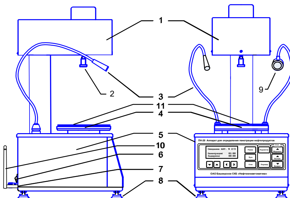
Рисунок 1 – Устройство пенетрометра
